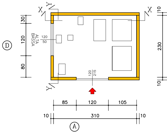
PIANTA CABINA
