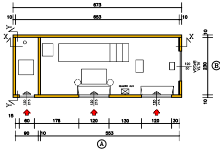
PIANTA CABINA
