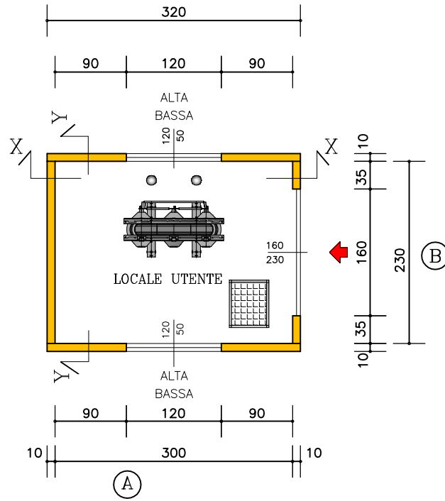
PIANTA CABINA
