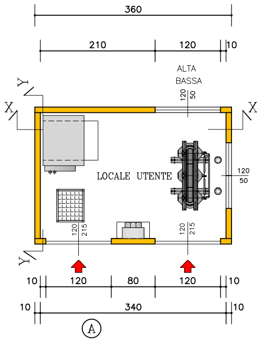
PIANTA CABINA
