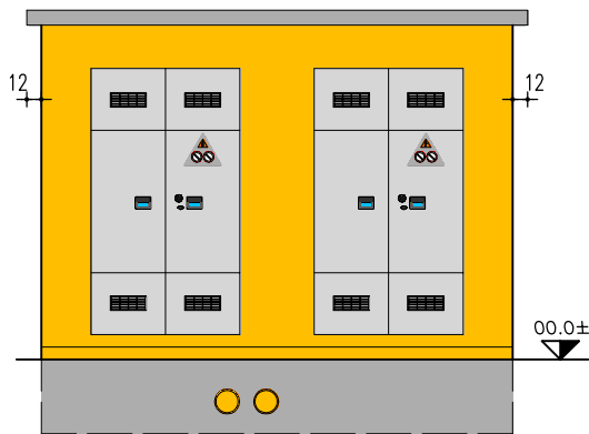
PROSPETTO A
