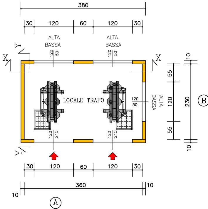
PIANTA CABINA
