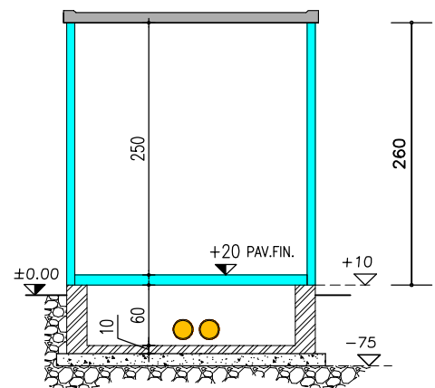
SEZIONE Y-Y
