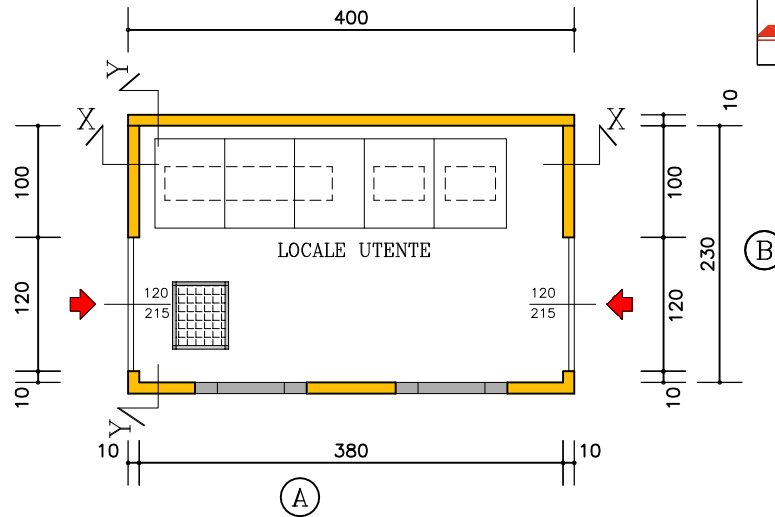
PIANTA CABINA
