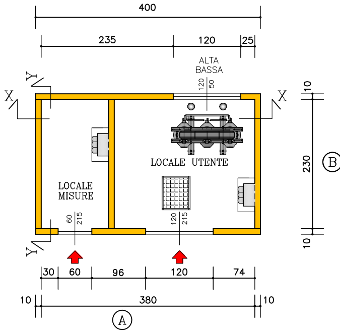
PIANTA CABINA
