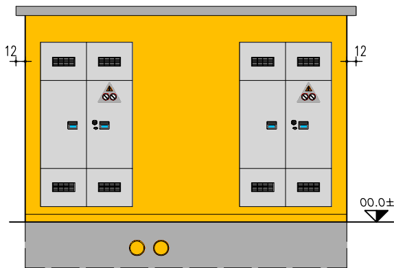
PROSPETTO A
