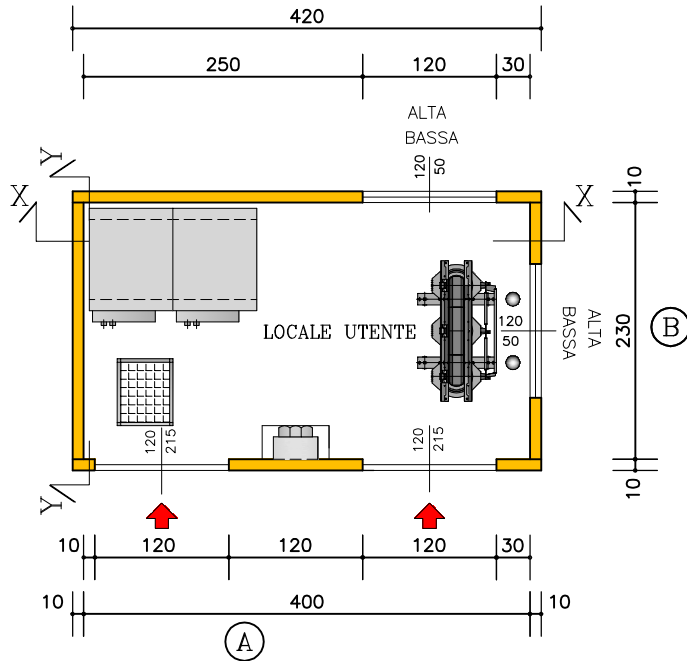
PIANTA CABINA
