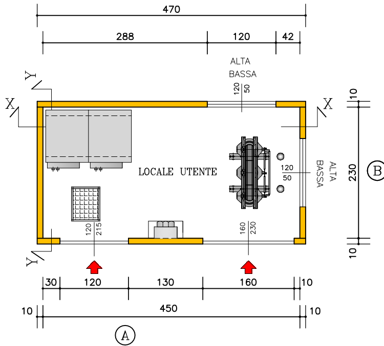
PIANTA CABINA
