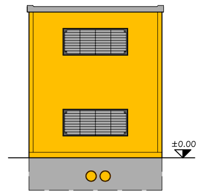
PROSPETTO B
