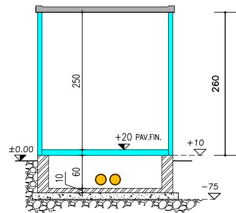
SEZIONE Y-Y
