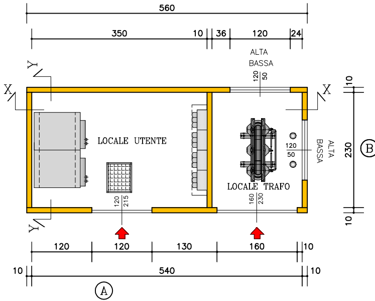
PIANTA CABINA
