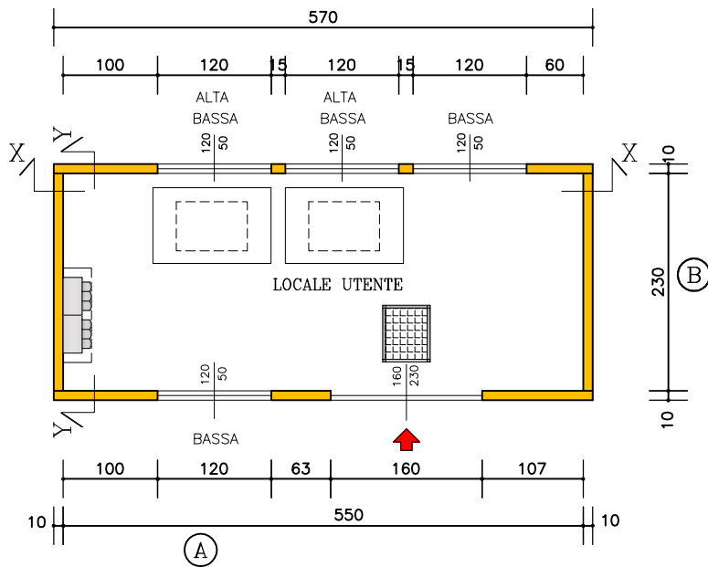
PIANTA CABINA
