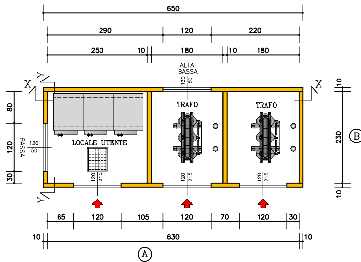
PIANTA CABINA
