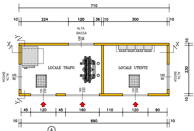
PIANTA CABINA
