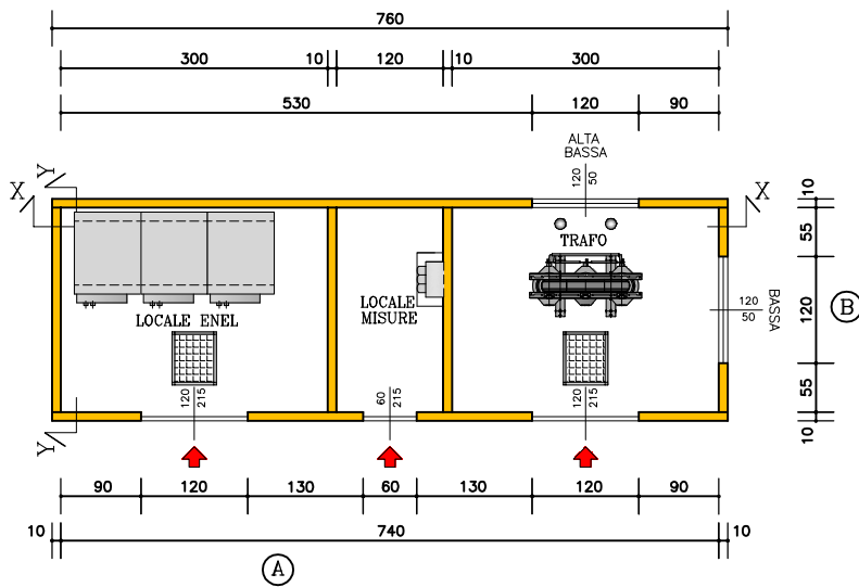
PIANTA CABINA
