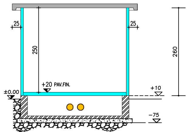
SEZIONE Y-Y
