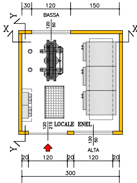
(A) PIANTA CABINA
