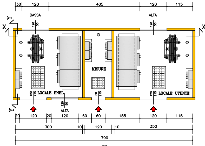
PIANTA CABINA
