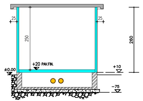
SEZIONE Y-Y
