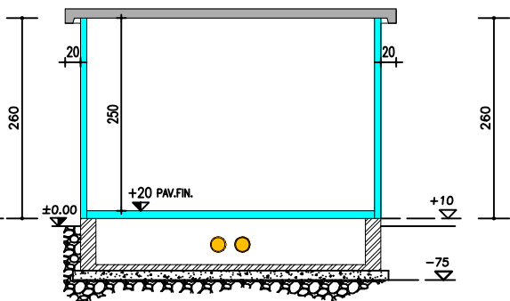
SEZIONE Y-Y
