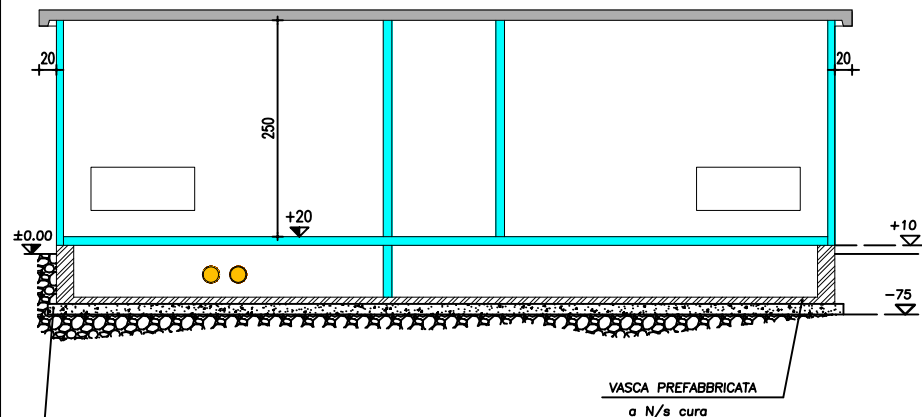
PROSPETTO A
