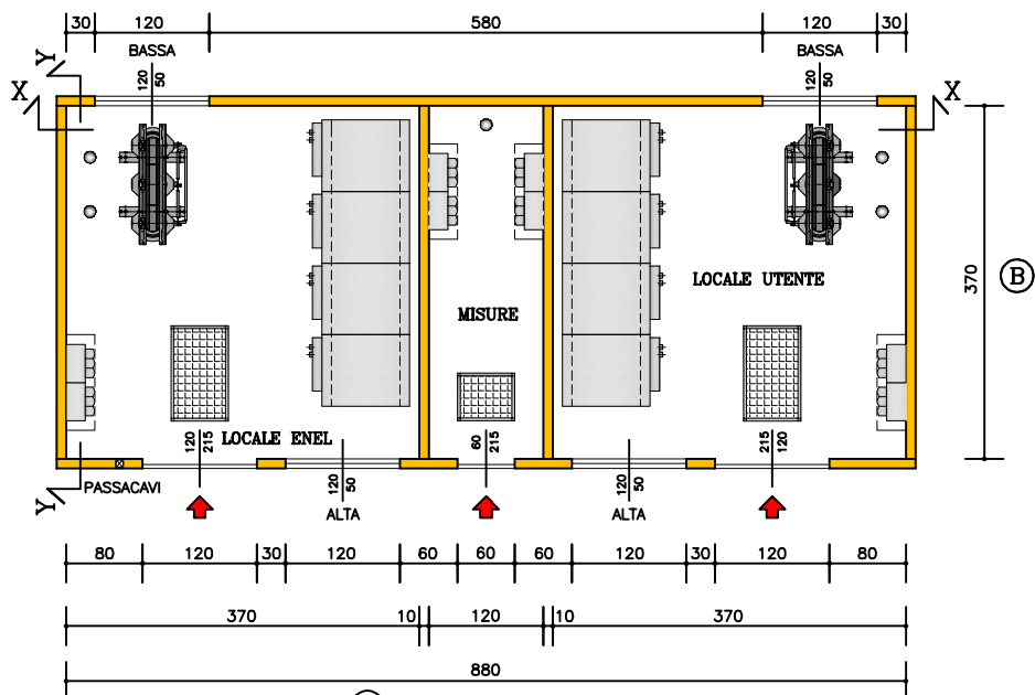
PIANTA CABINA
