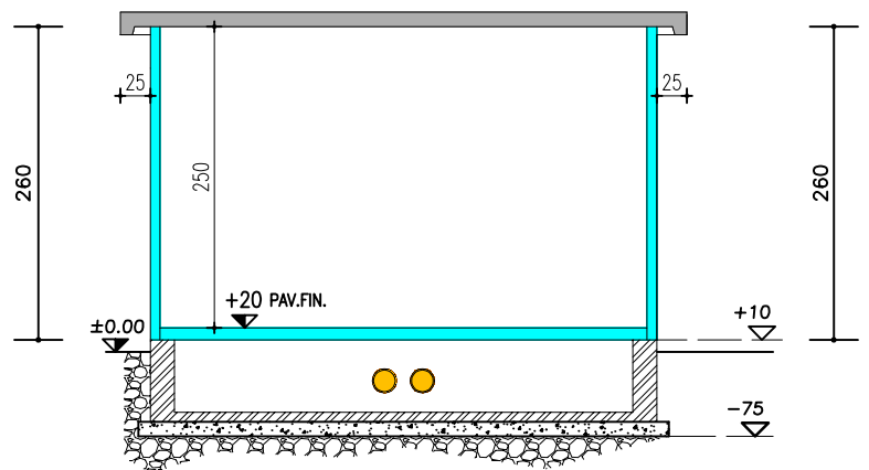
SEZIONE Y-Y
