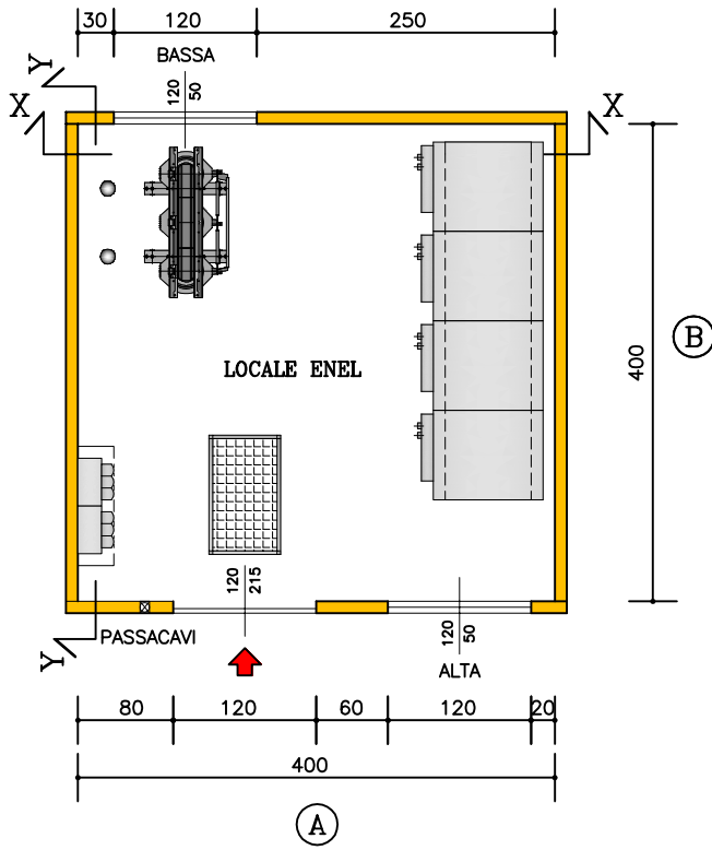
PIANTA CABINA
