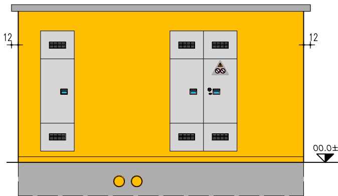
PROSPETTO A
