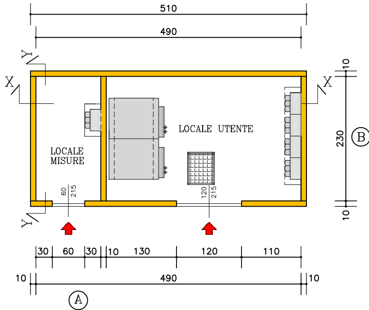
PIANTA CABINA
