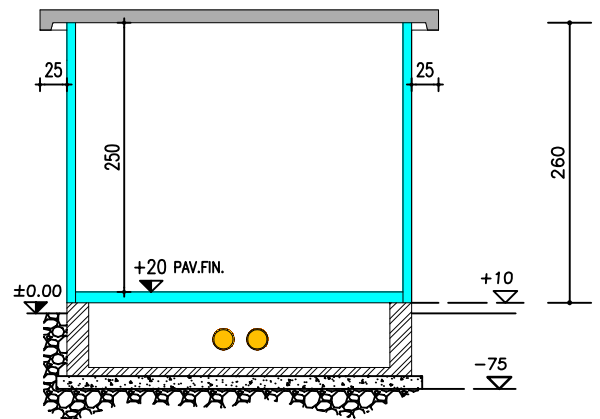
SEZIONE Y-Y
