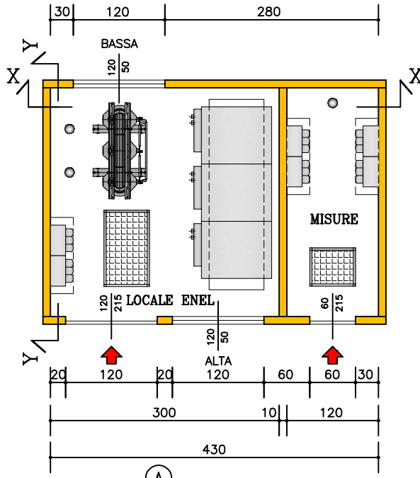
PIANTA CABINA
