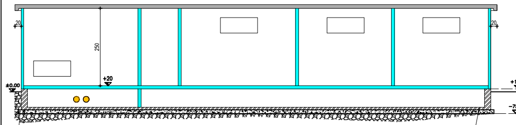
PROSPETTO A
