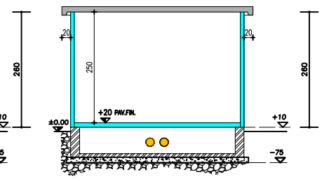
SEZIONE Y-Y
