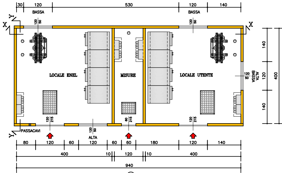
PIANTA CABINA
