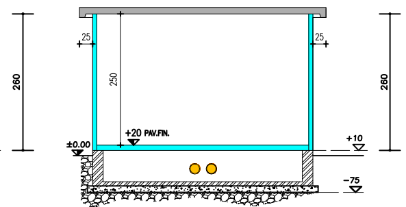
SEZIONE Y-Y
