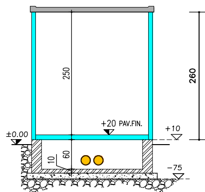
SEZIONE X-X
