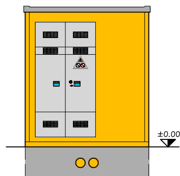
PROSPETTO B
