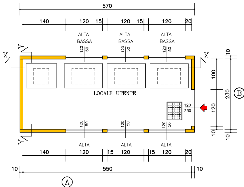
PIANTA CABINA
